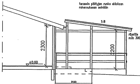
Leikkaus
